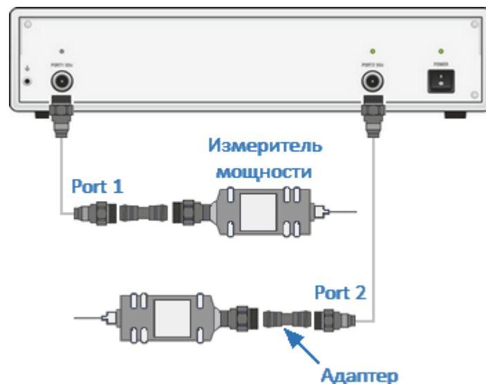
Рисунок 153 – Калибровка мощности с помощью внешнего измерителя мощности
