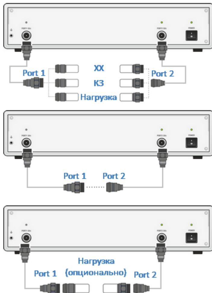
Рисунок 135 – Полная двухпортовая калибровка
