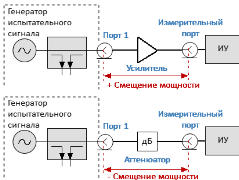
Рисунок 63 – Смещение мощности порта
