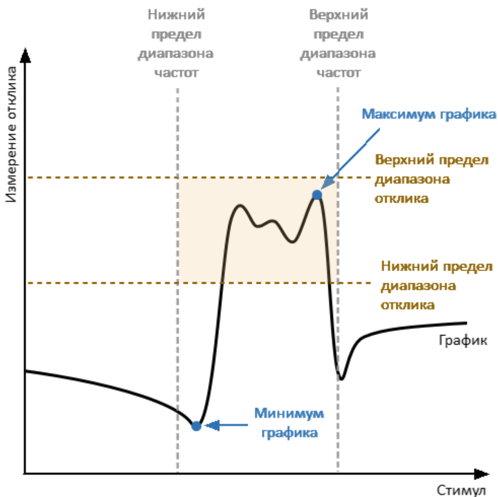
Рисунок 205 – Тест пределов для пика
