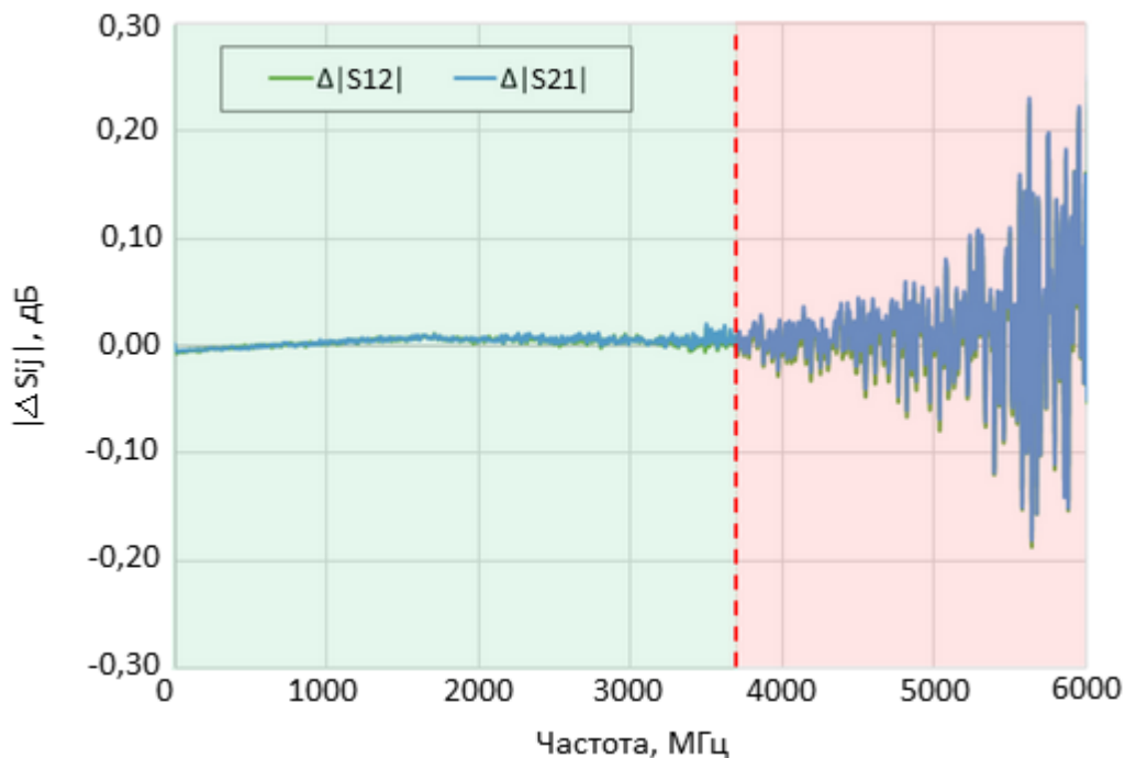
Рисунок 170 – Отклонение коэффициента передачи \Delta|S_{ij}| = |S_{ii}^{ACMB} - S_{ii}^{BAЦ}|
