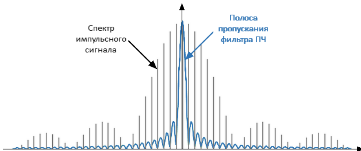
Рисунок 249 – Узкополосное детектирование
