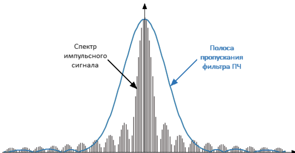
Рисунок 248 – Широкополосное детектирование
