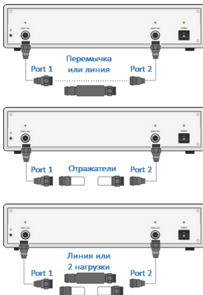
Рисунок 149 – Калибровка TRL
