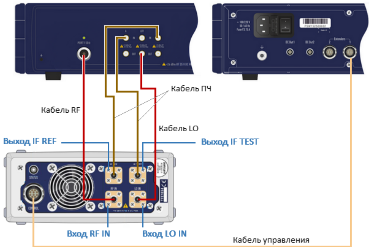
Рисунок 227 – Схема подключения модуля TFE-1854 к анализатору
