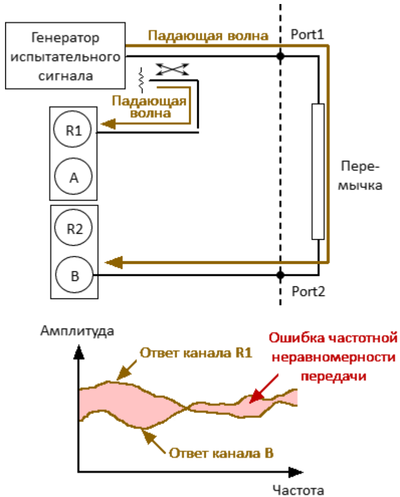
Рисунок 116 – Ошибка частотной неравномерности передачи
