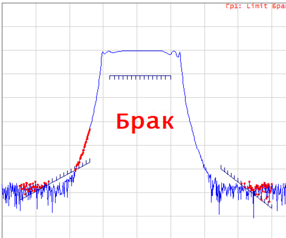
Рисунок 199 – Пример отрицательных результатов допускового контроля
