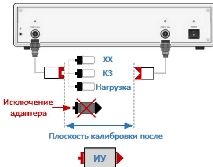
Рисунок 146 – Второй этап функции исключения адаптера
