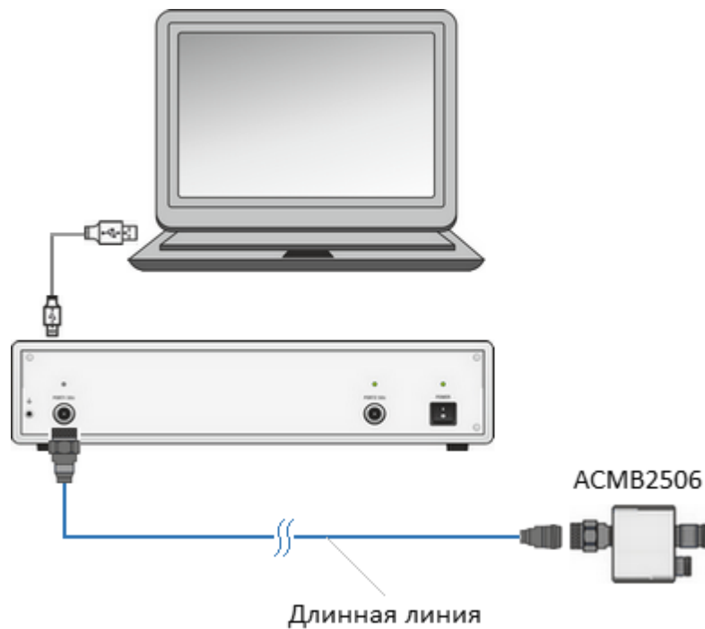
Рисунок 164 – Схема измерения S-параметров длинной линии с помощью АСМВ2506
