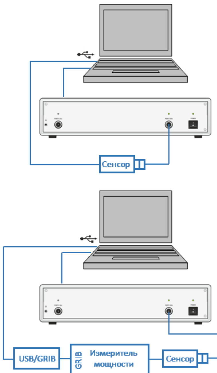
Рисунок 263 – Пример подключения измерителя мощности
