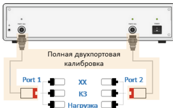
Рисунок 141 – Первый этап калибровки с неизвестной перемычкой SOLR
