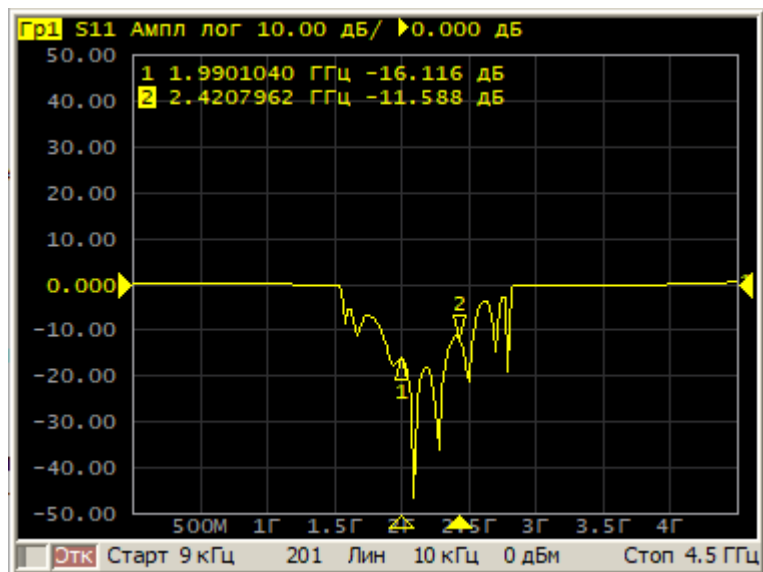
Рисунок 264 – Нет секретности
