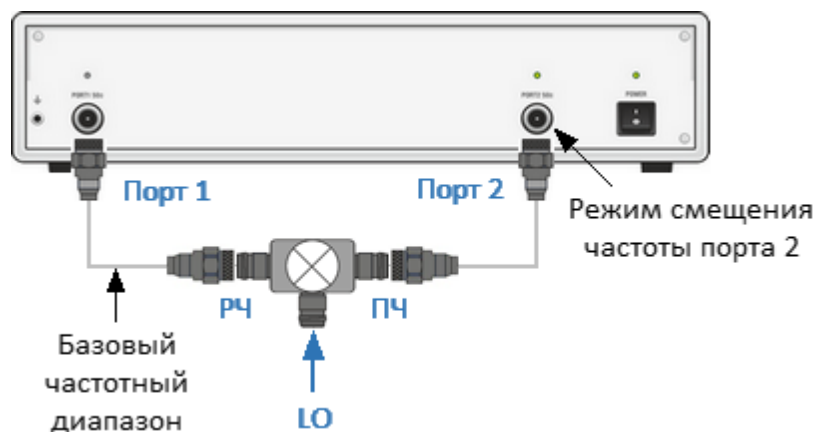
Рисунок 215 – Измерение смесителя с использованием смещения частоты
