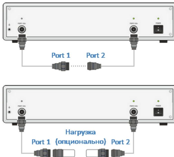
Рисунок 132 – Калибровка нормализации передачи
