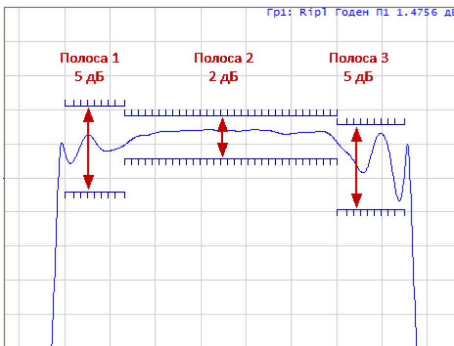
Рисунок 201 – Пример пределов пульсаций
