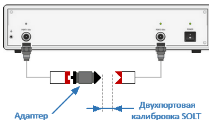
Рисунок 145 – Первый этап функции исключения адаптера
