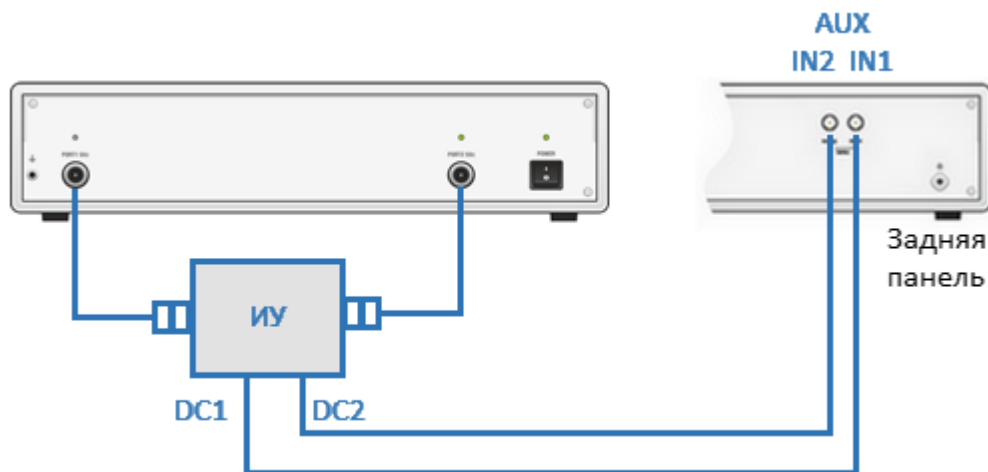
Рисунок 230 – Пример схемы подключения ИУ к вольтметру
