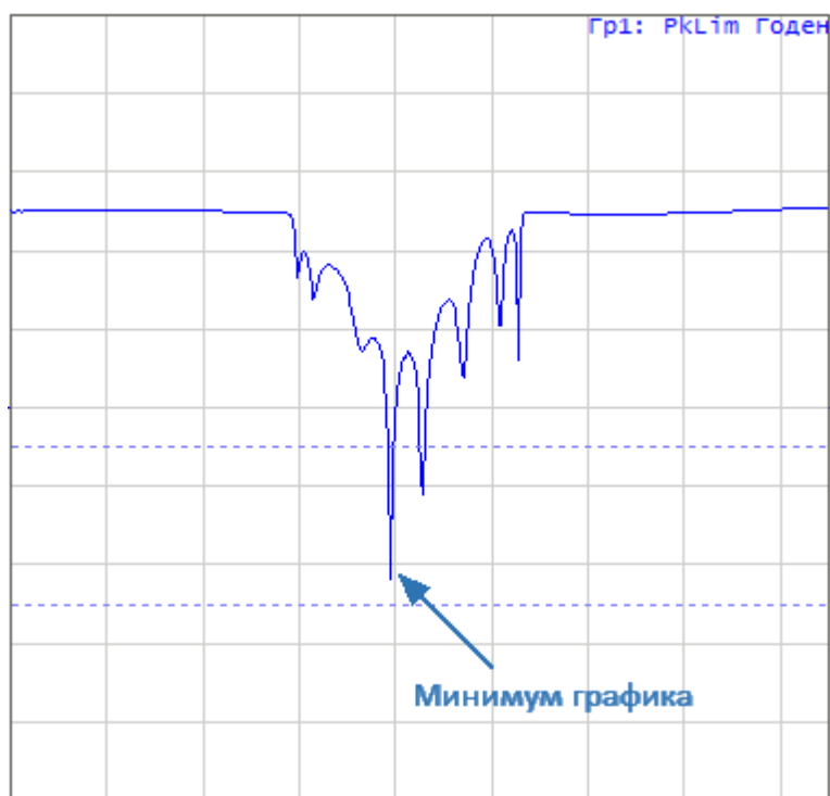
Рисунок 206 – Пример пройденного теста (Тип предела: "Отклик")
