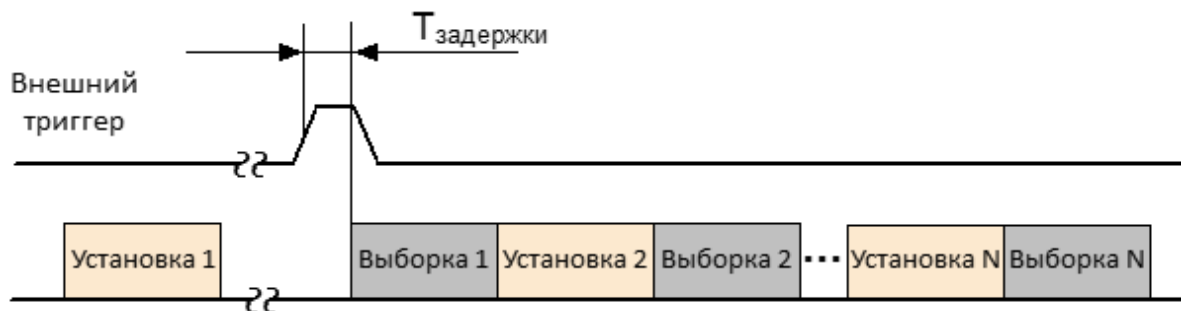
Рисунок 68 — Задержка внешнего триггера
