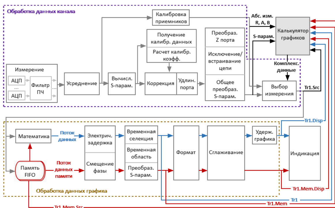
Рисунок 209 – Блок-схема конвейера обработки данных
