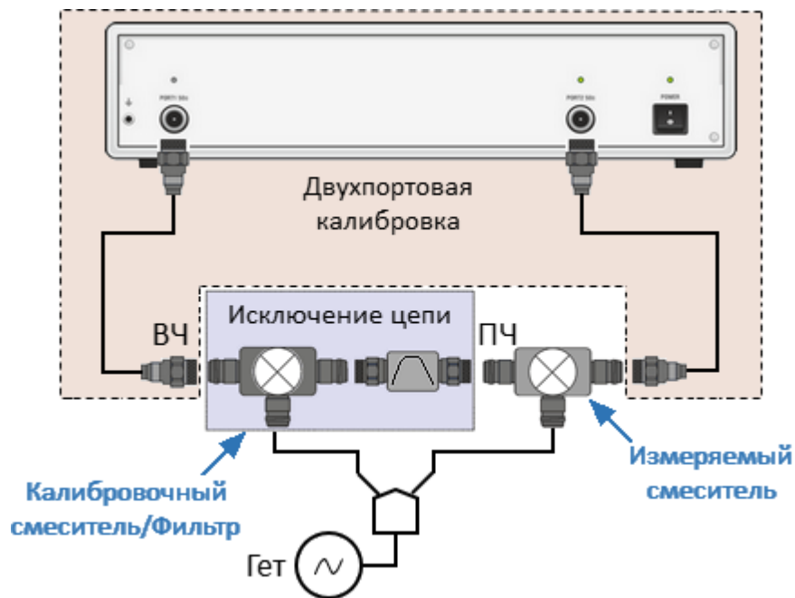
Рисунок 157 – Векторные измерения смесителей
