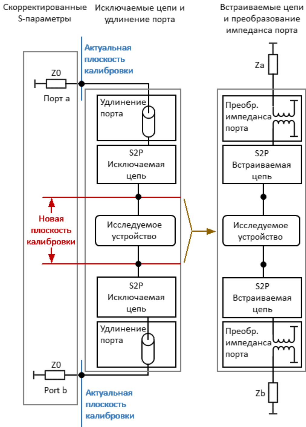
Рисунок 190 – Логическая схема функции моделирования оснастки
