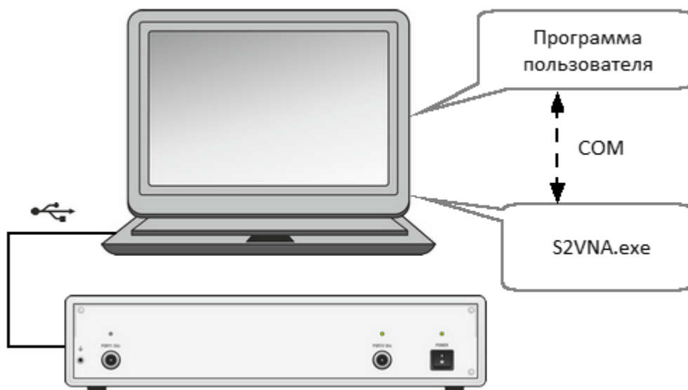
Рисунок 281 – Технология COM
