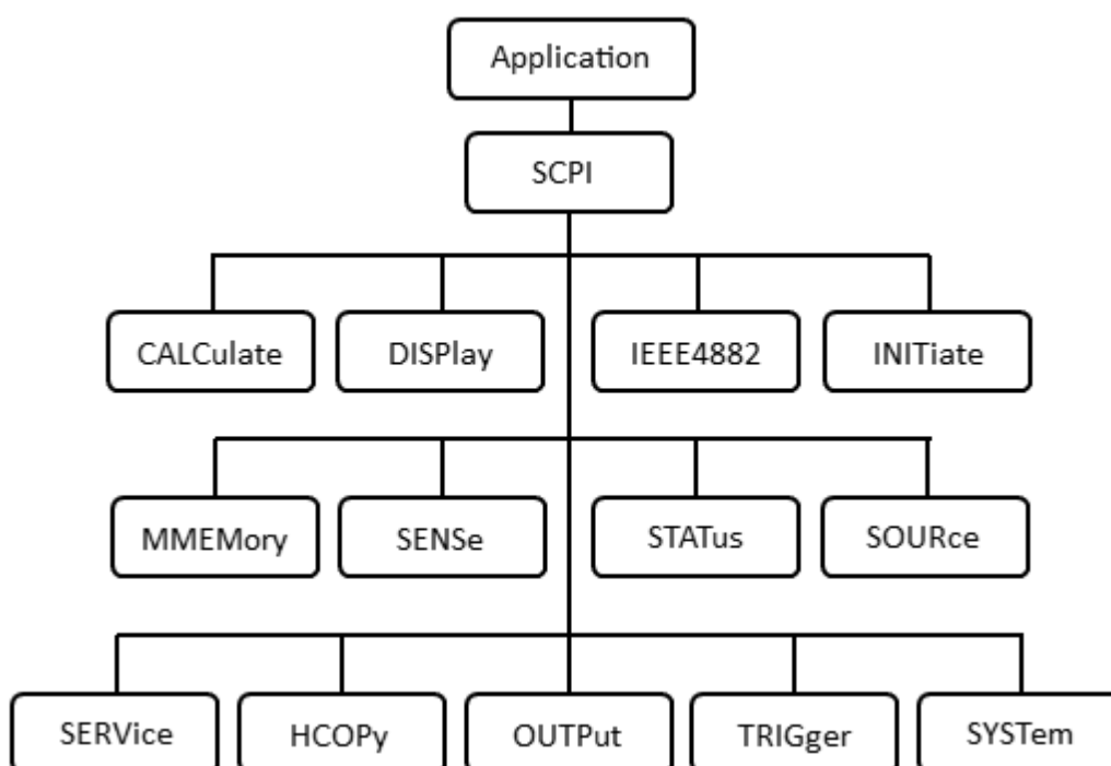
Рисунок 283 –Структура COM-объектов
