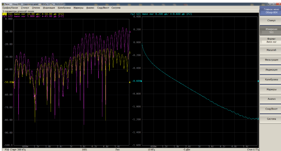
Рисунок 167 – Пример графиков S-параметров длинной линии, измеренных с помощью АСМВ2506
