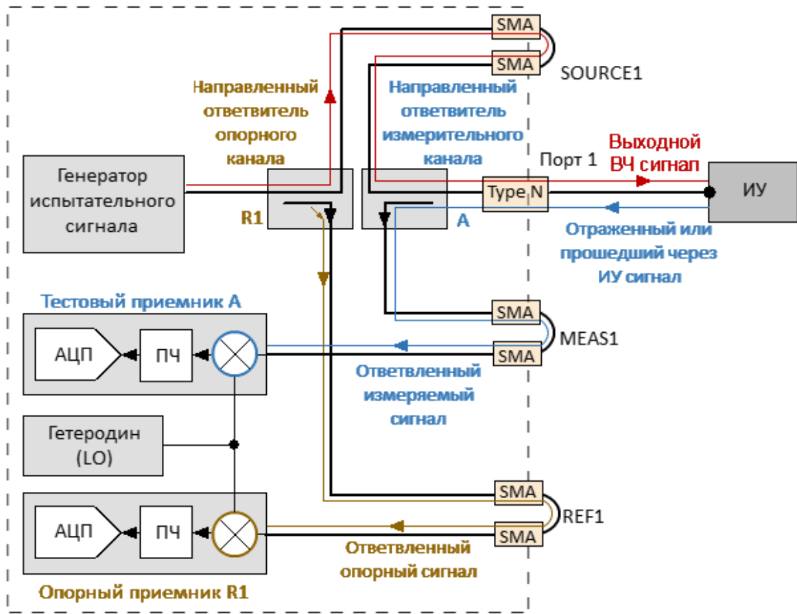
Рисунок 231 – Анализатор C2209, распространение сигнала в общем режиме
