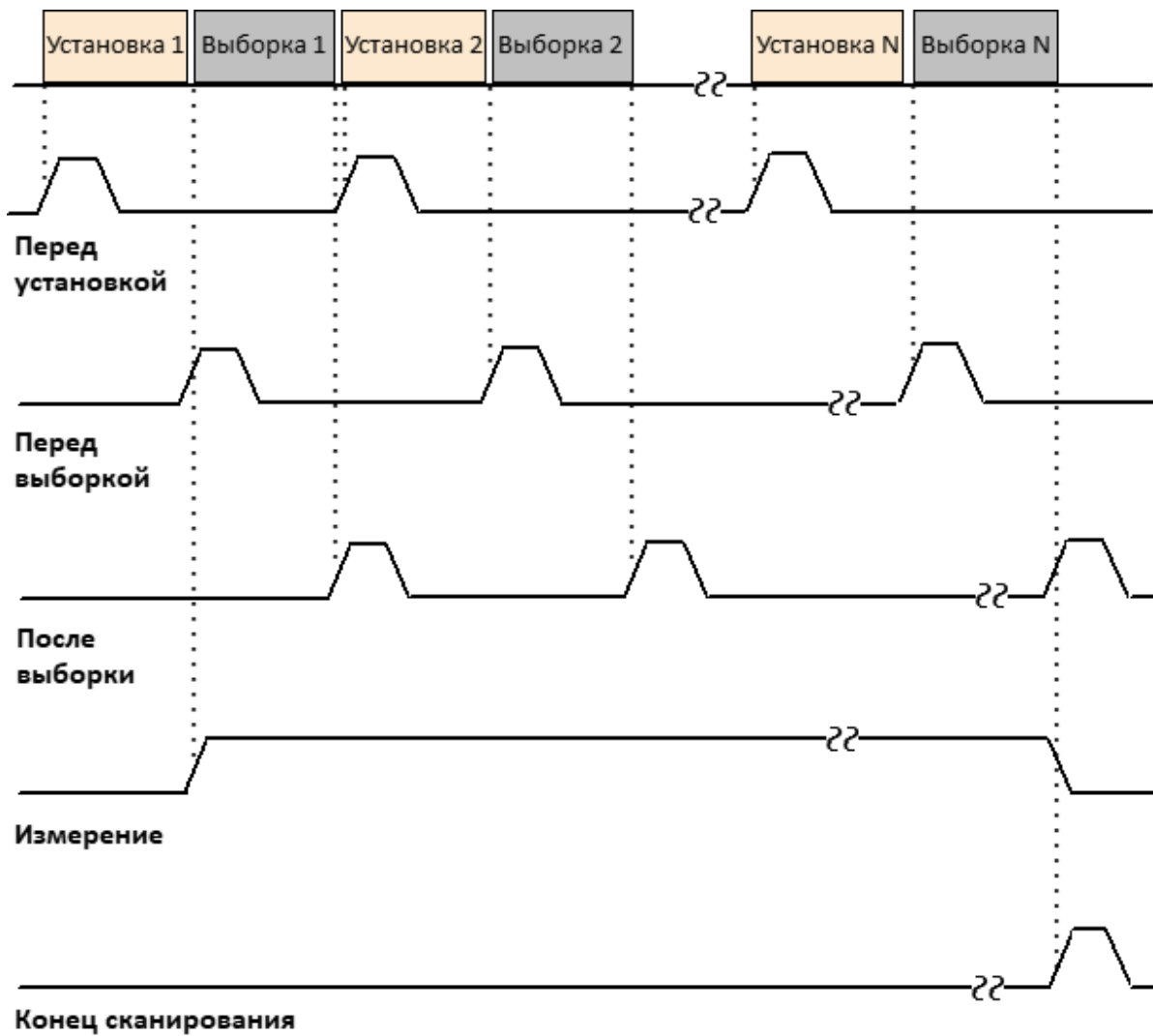
Рисунок 70 — Выходной сигнала триггера (за исключением "готов к триггеру")
