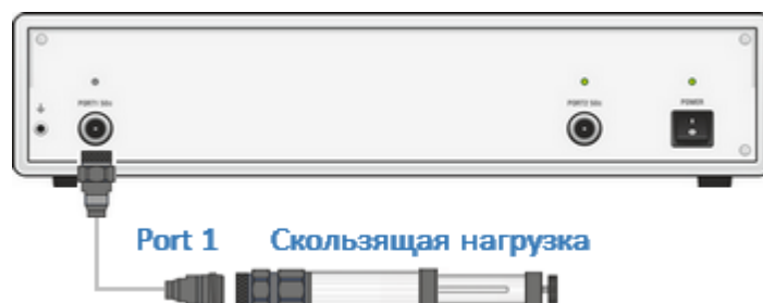
Рисунок 136 – Калибровка скользящей нагрузкой
