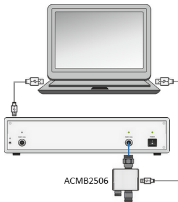
Рисунок 163 – Схема подключения ACMB2506 для калибровки и настройки
