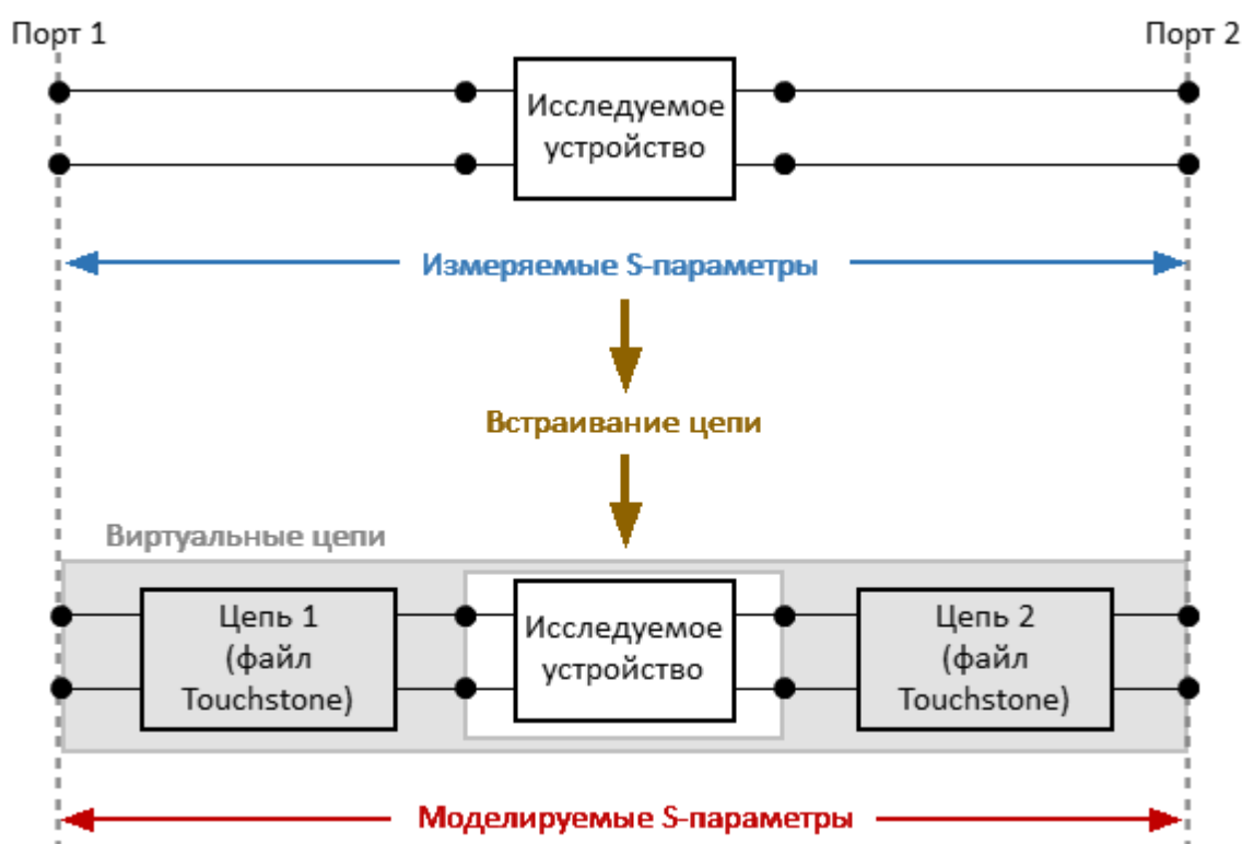
Рисунок 196 – Встраивание цепи
