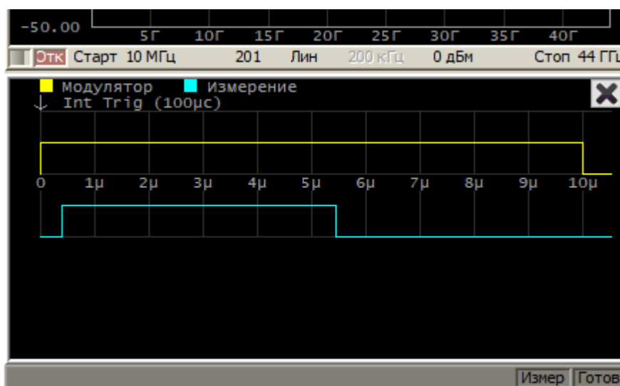
Рисунок 253 – Пример временной диаграммы для настройки импульсного режима
