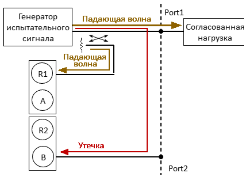
Рисунок 117 – Ошибка развязки
