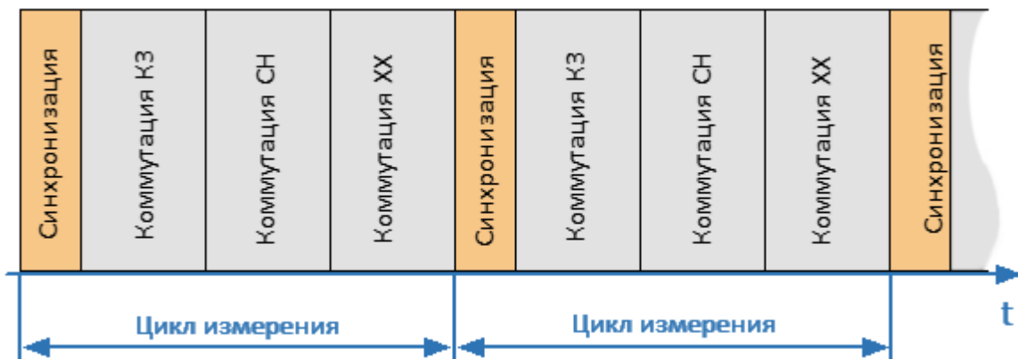
Рисунок 162 – Временная диаграмма рабочего цикла модуля
