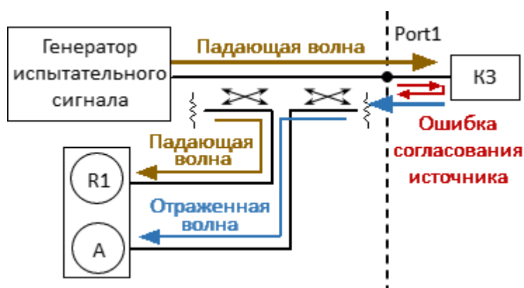
Рисунок 113 – Ошибка согласования источника
