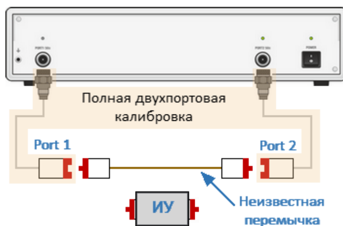
Рисунок 142 – Второй этап калибровки с неизвестной перемычкой SOLR
