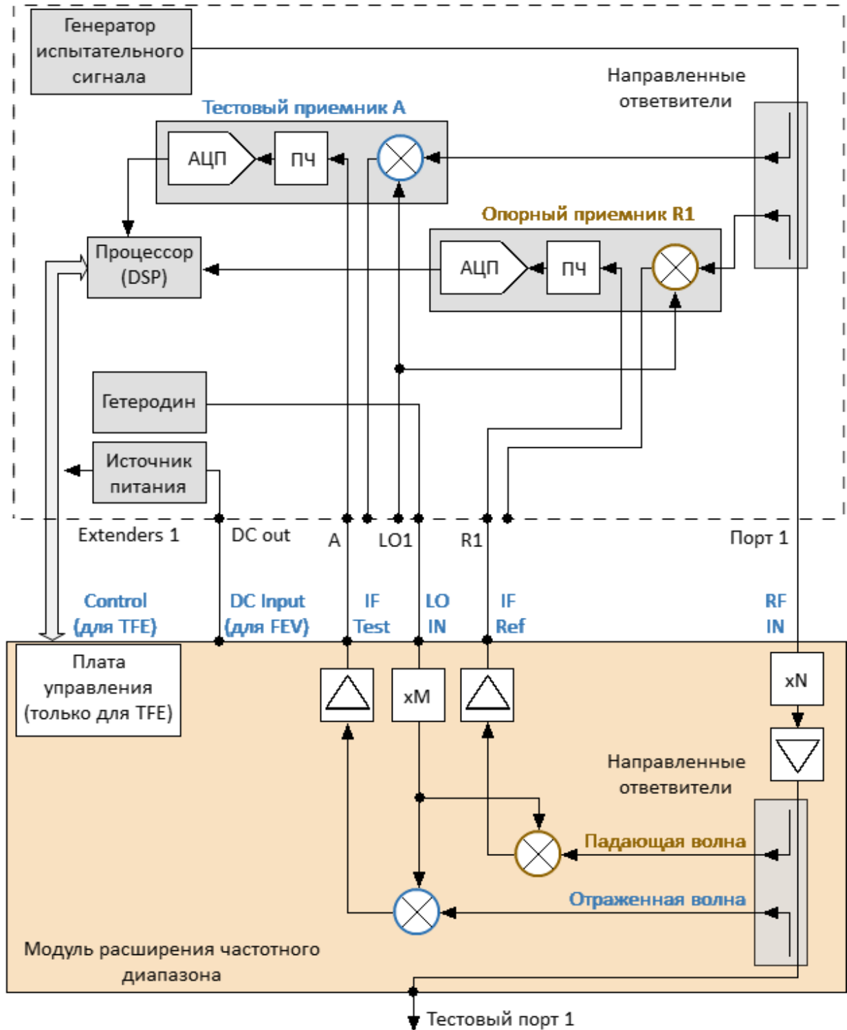
Рисунок 223 – Структурная схема подключения модуля к анализатору
