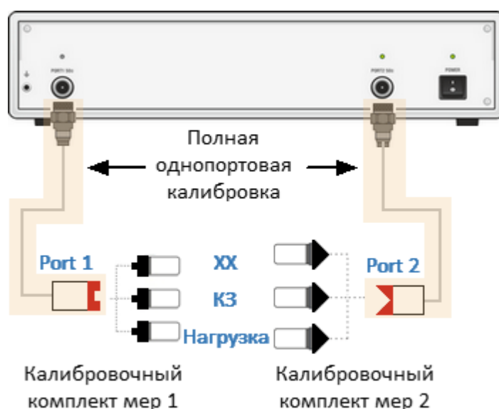
Рисунок 143 – Однопортовая калибровка перед добавлением неизвестной перемычки
