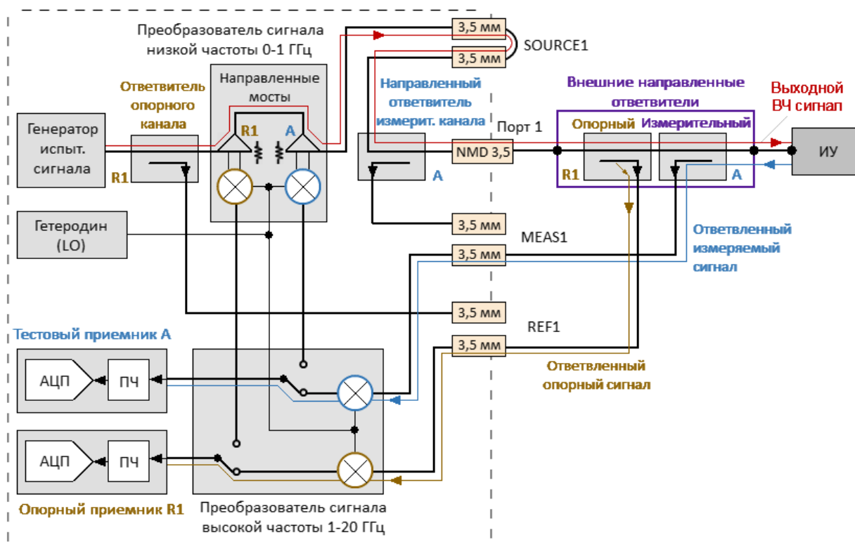
Рисунок 235 – Анализатор C2220, распространение сигнала в режиме прямого доступа
