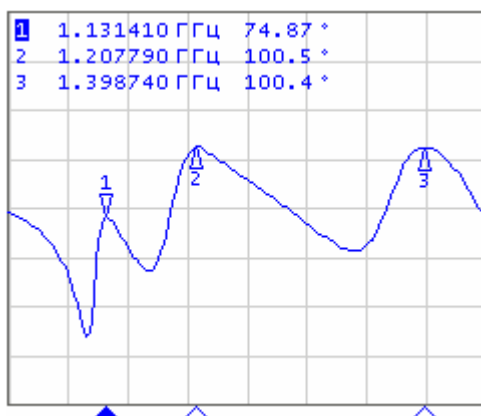
Рисунок 182 – Пример положительных пиков
