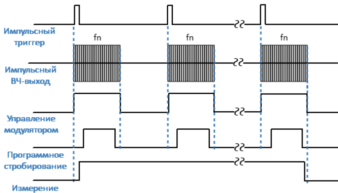
Рисунок 257 – Измерение в одной точке развертки в узкополосном режиме
