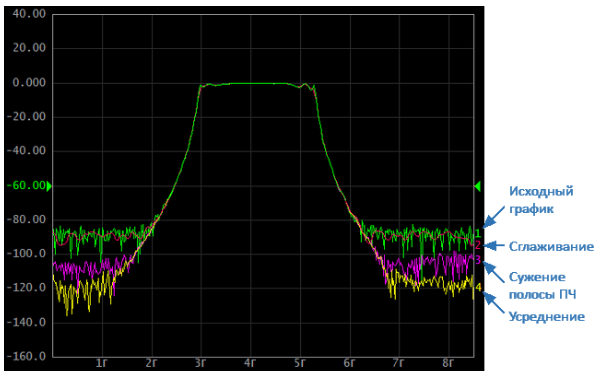
Рисунок 82 — Сравнение методов фильтрации
