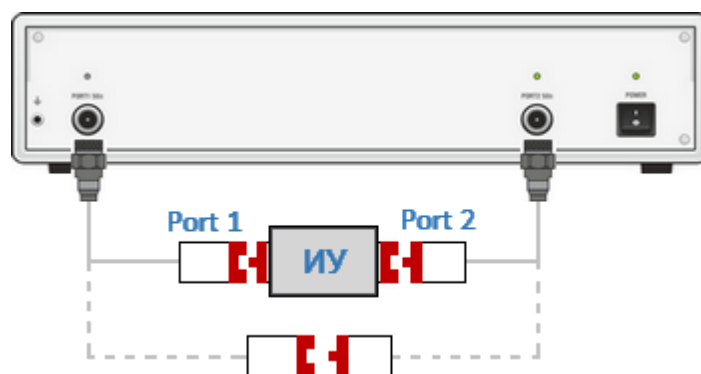
Рисунок 138 – Пример устройства с присоединяемыми портами
