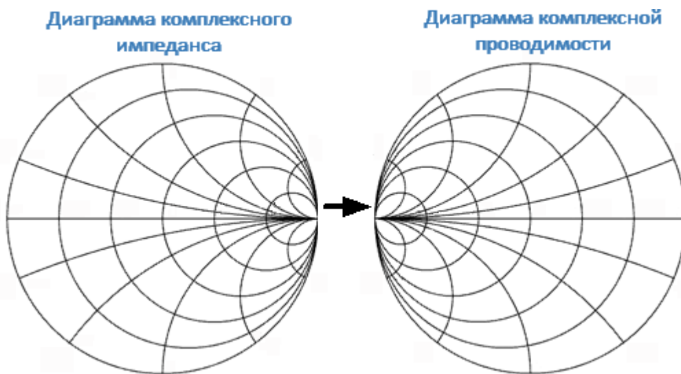
Рисунок 79 — Преобразование диаграммы комплексного импеданса в диаграмму комплексной проводимости
