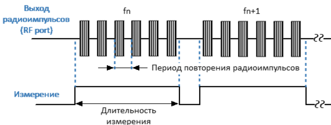
Рисунок 256 – Формирование развертки в узкополосном режиме
