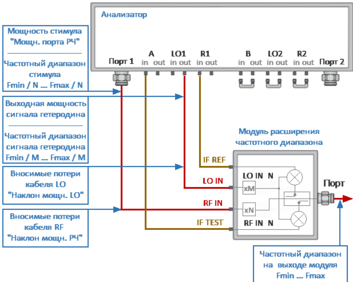
Рисунок 229 – Схема установки параметров модуля
