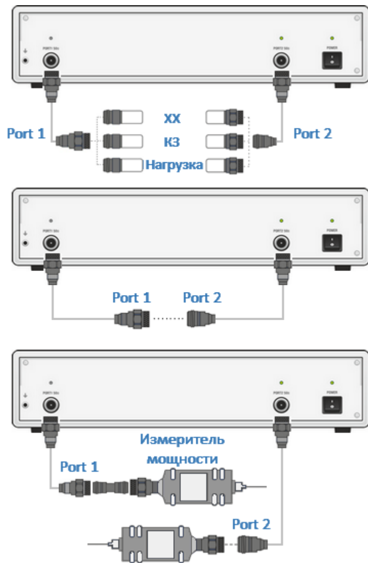
Рисунок 156 – Схема скалярной калибровки смесителей
