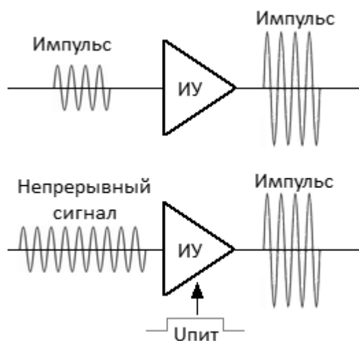
Рисунок 237 – Принцип измерения импульсных устройств
