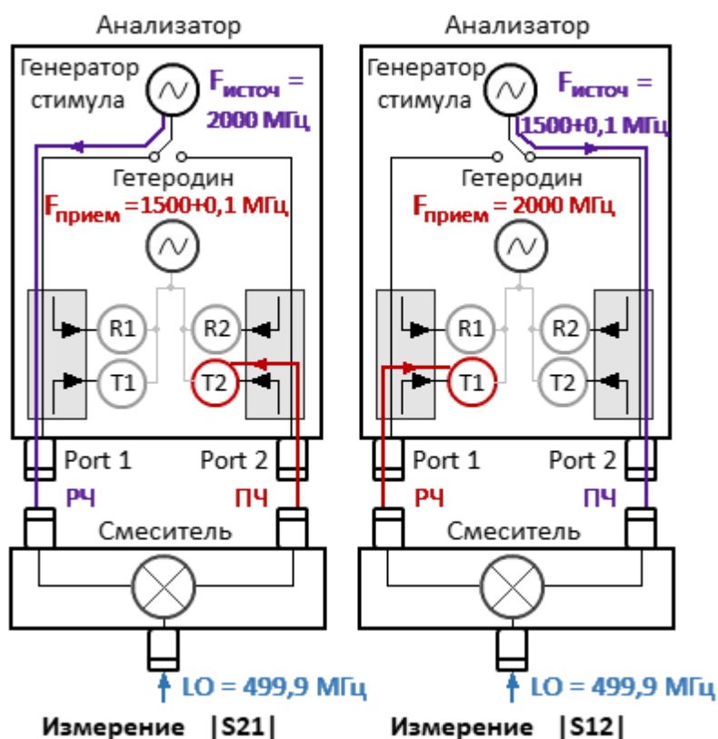
Рисунок 222 — Измерение коэффициента передачи смесителя в режиме АПЧС с подстройкой частоты порта 2
