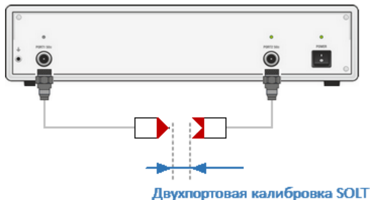
Рисунок 147 – Первый этап функции добавления адаптера
