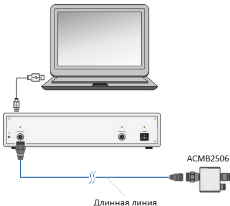
Рисунок 161 – Подключение АСМВ2506 в режиме измерения длинной линии
