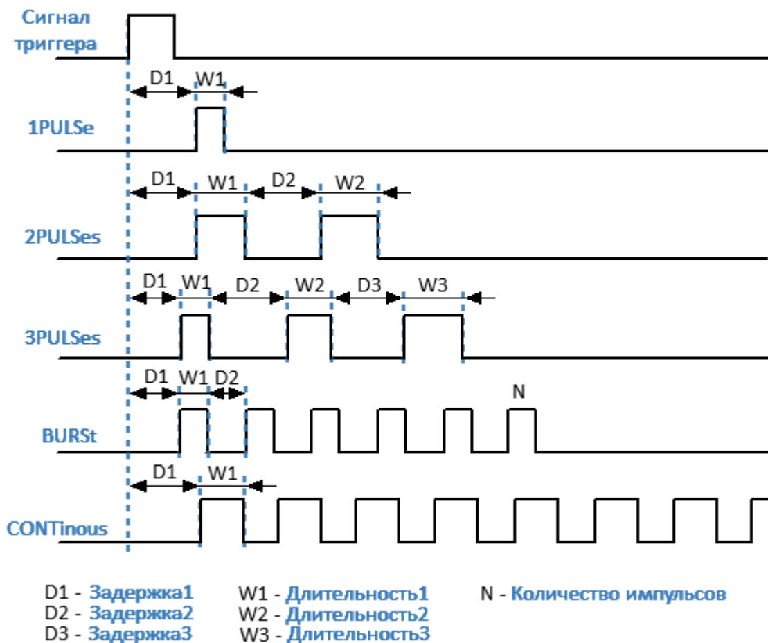
Рисунок 286 – Временная диаграмма настроек импульсного генератора
