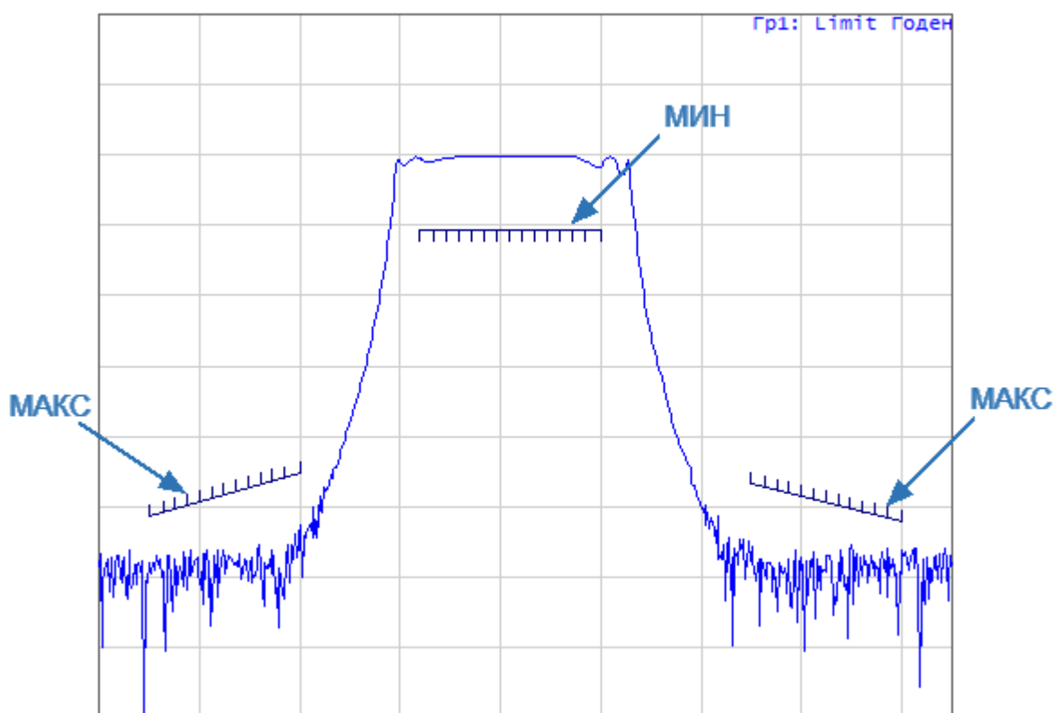
Рисунок 198 – Пример линии пределов
