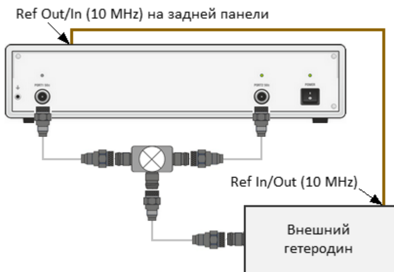
Рисунок 218 — Синхронизация анализатора и внешнего гетеродина по опорной частоте
