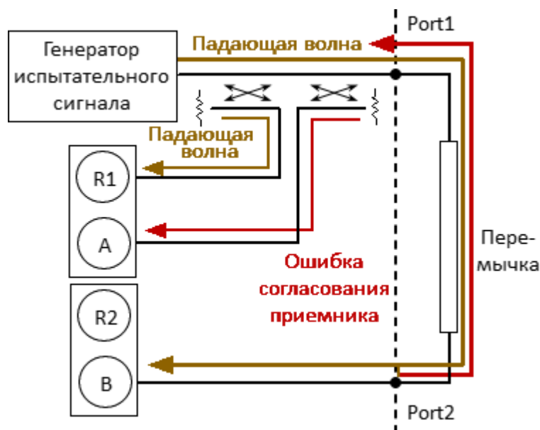
Рисунок 114 – Ошибка согласования приемника
