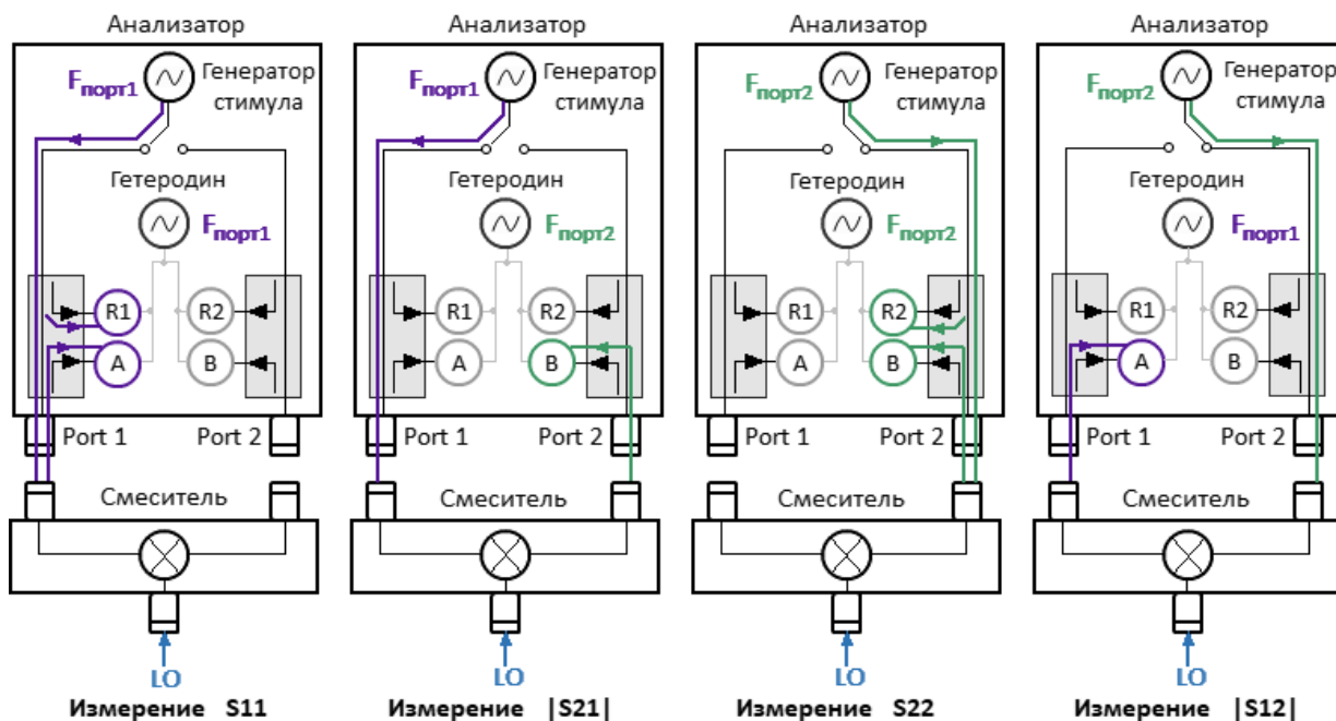
Рисунок 214 — Измерение матрицы S-параметров в режиме смещения частоты между портами
