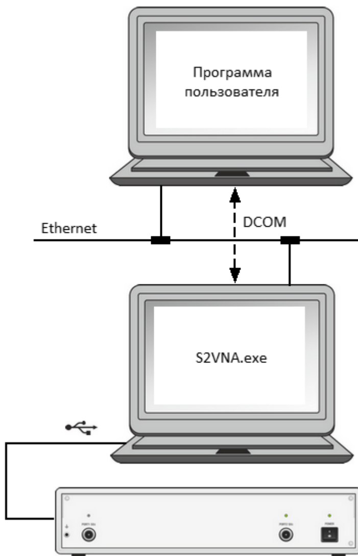
Рисунок 282 – Технология DCOM
