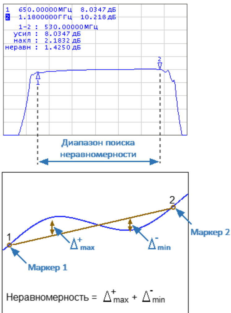
Рисунок 187 – Поиск неравномерности
