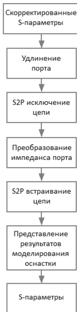
Рисунок 191 – Блок-схема обработки данных при моделировании оснастки
