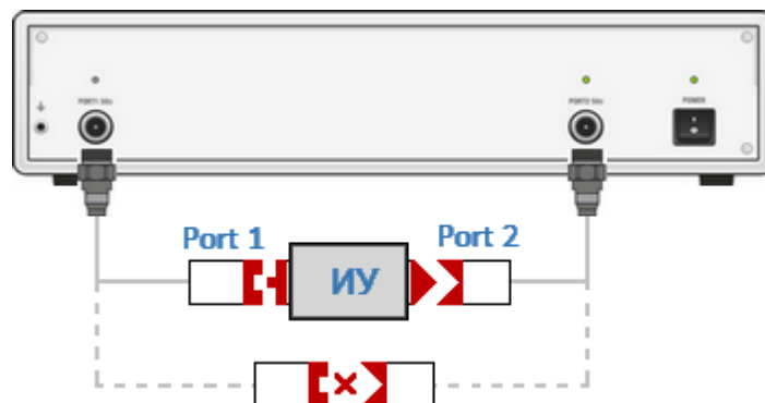
Рисунок 140 – Пример устройства с не присоединяемыми портами (соединители имеют разный тип разъемов)
