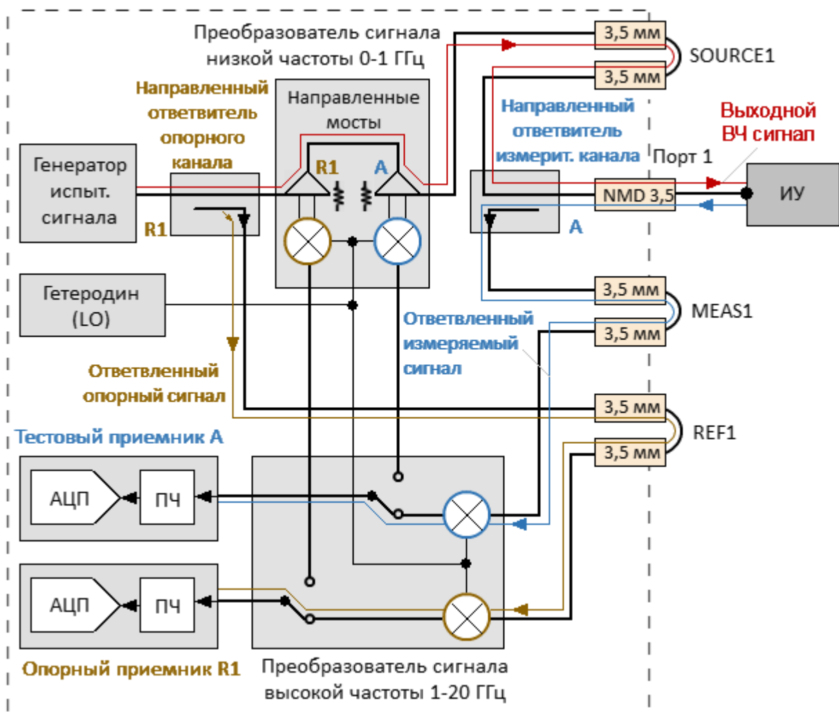
Рисунок 234 – Анализатор С2220, распространение сигнала в общем режиме (диапазон от 1 до 20 ГГц)
