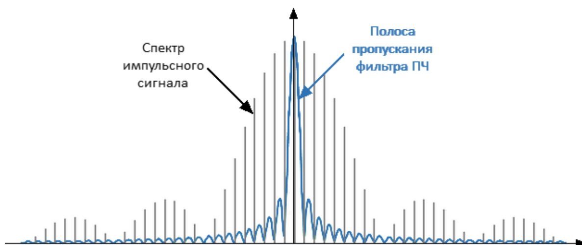
Рисунок 239 – Узкополосное детектирование
