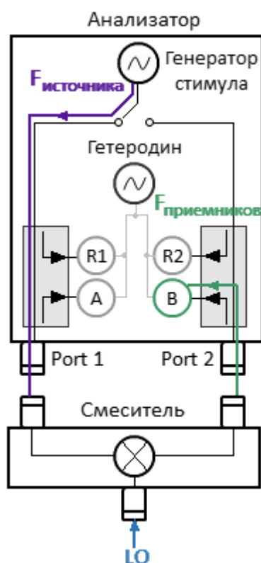
Рисунок 217 — Измерение смесителя в режиме смещения частоты "источник/приёмник"
