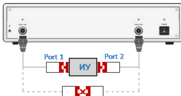
Рисунок 139 – Пример устройства с не присоединяемыми портами (соединители одного типа)
