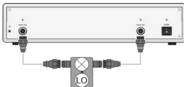
Рисунок 219 — Измерение смесителя со встроенным гетеродином (синхронизация невозможна)
