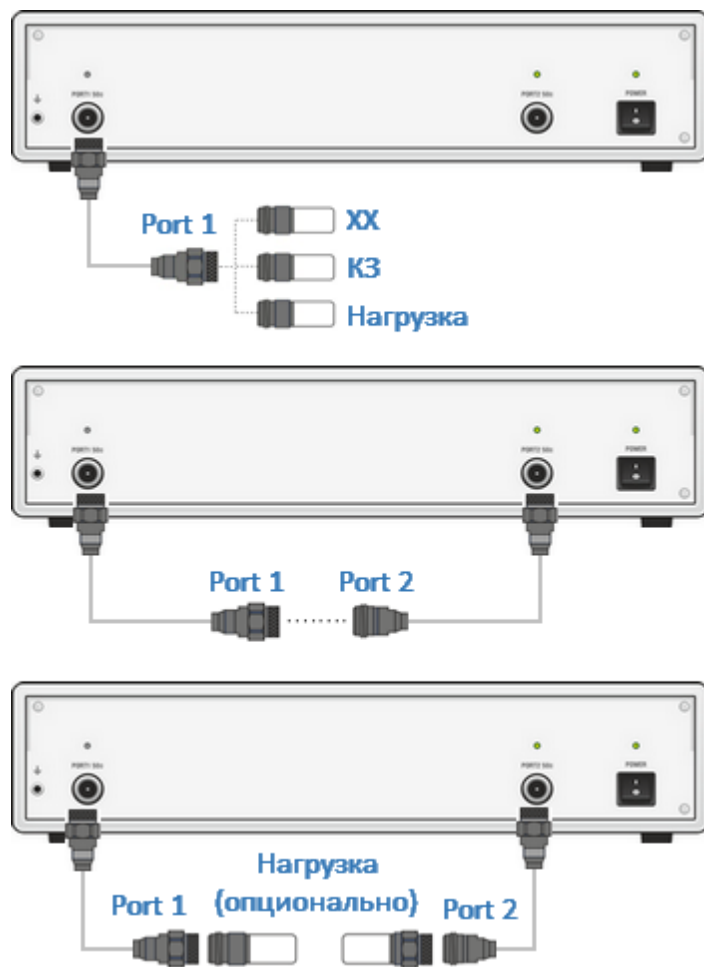
Рисунок 134 – Однонаправленная двухпортовая калибровка
