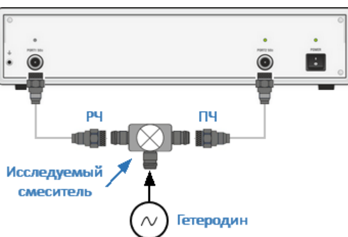
Рисунок 212 – Схема скалярного измерения смесителя
