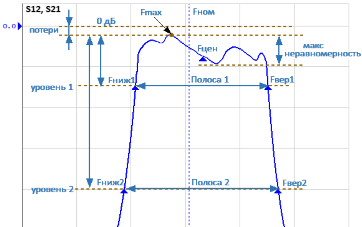
Рисунок 208 – Анализ полосно-пропускающего фильтра
