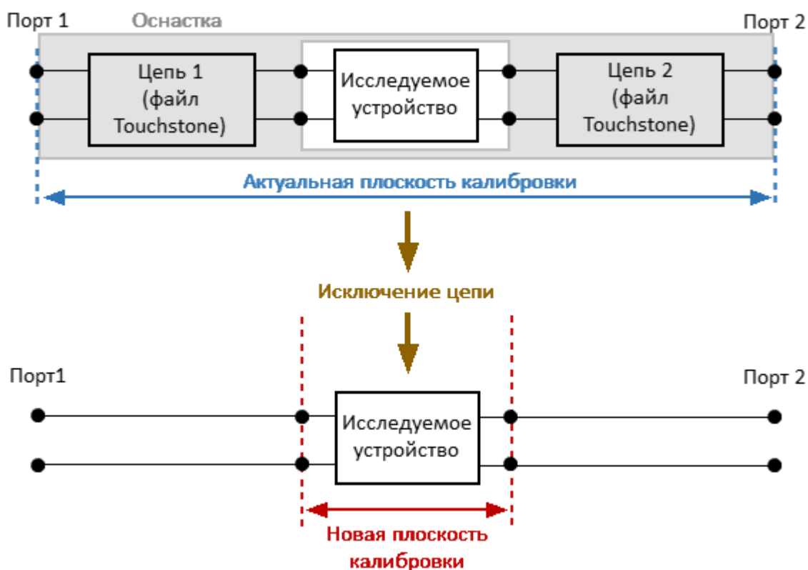
Рисунок 195 – Исключение цепи
