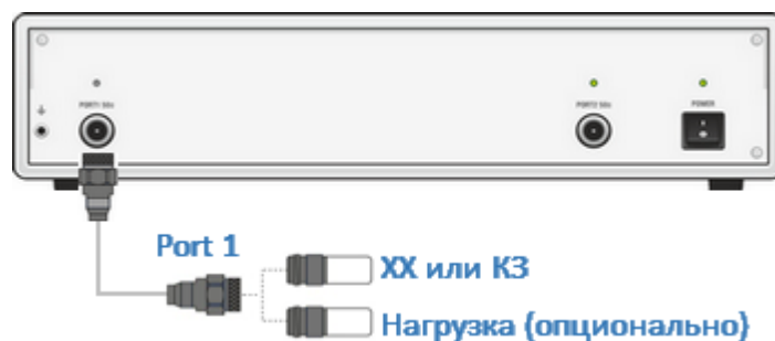
Рисунок 131 – Калибровка нормализации отражения
