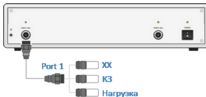
Рисунок 133 – Полная однопортовая калибровка
