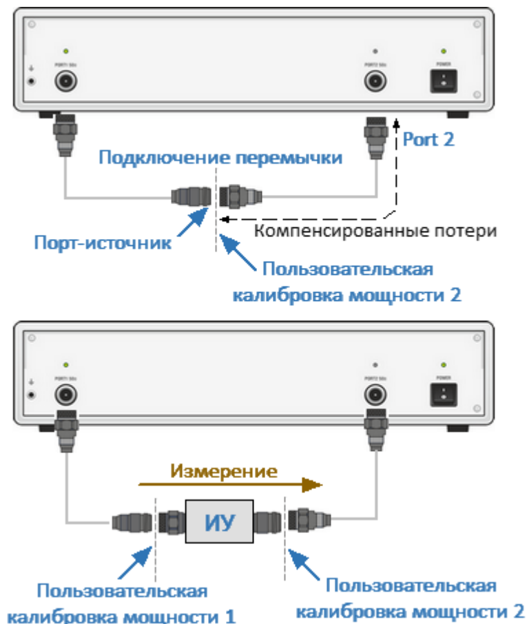
Рисунок 155 – Калибровка приемников
