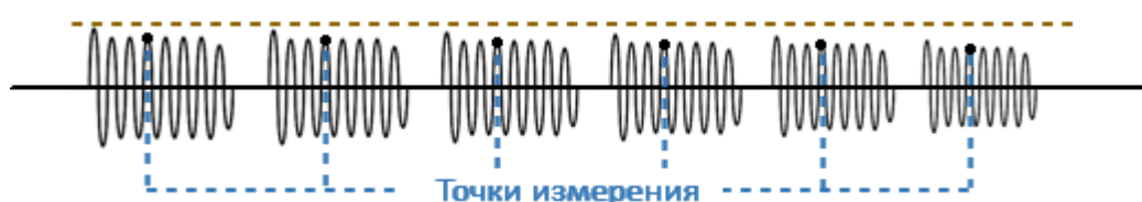
Рисунок 261 – Пример изменения коэффициента усиления от импульса к импульсу
