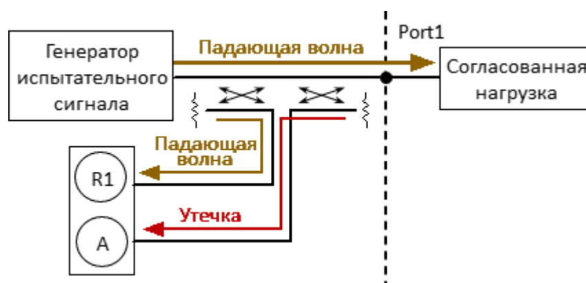
Рисунок 112 – Ошибка направленности
