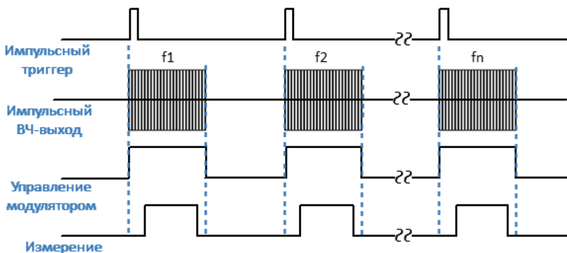
Рисунок 254 – Режим «Точка в импульсе»
