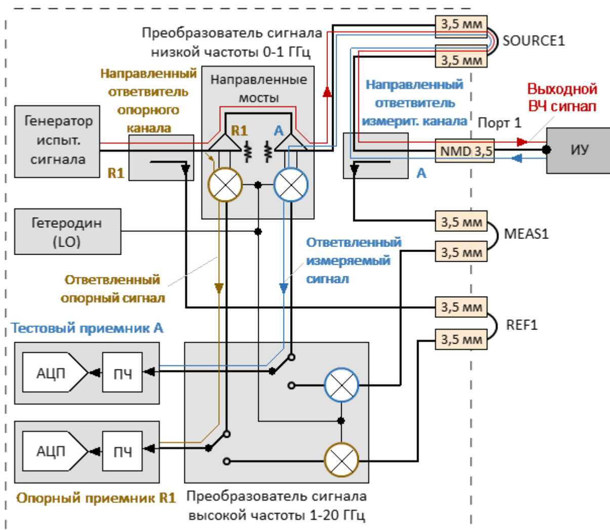
Рисунок 233 – Анализатор С2220, распространение сигнала в общем режиме (диапазон от 100 кГц до 1 ГГц)
