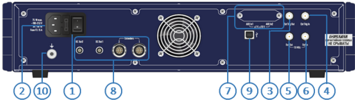
Рисунок 36 – Задняя панель С4209
