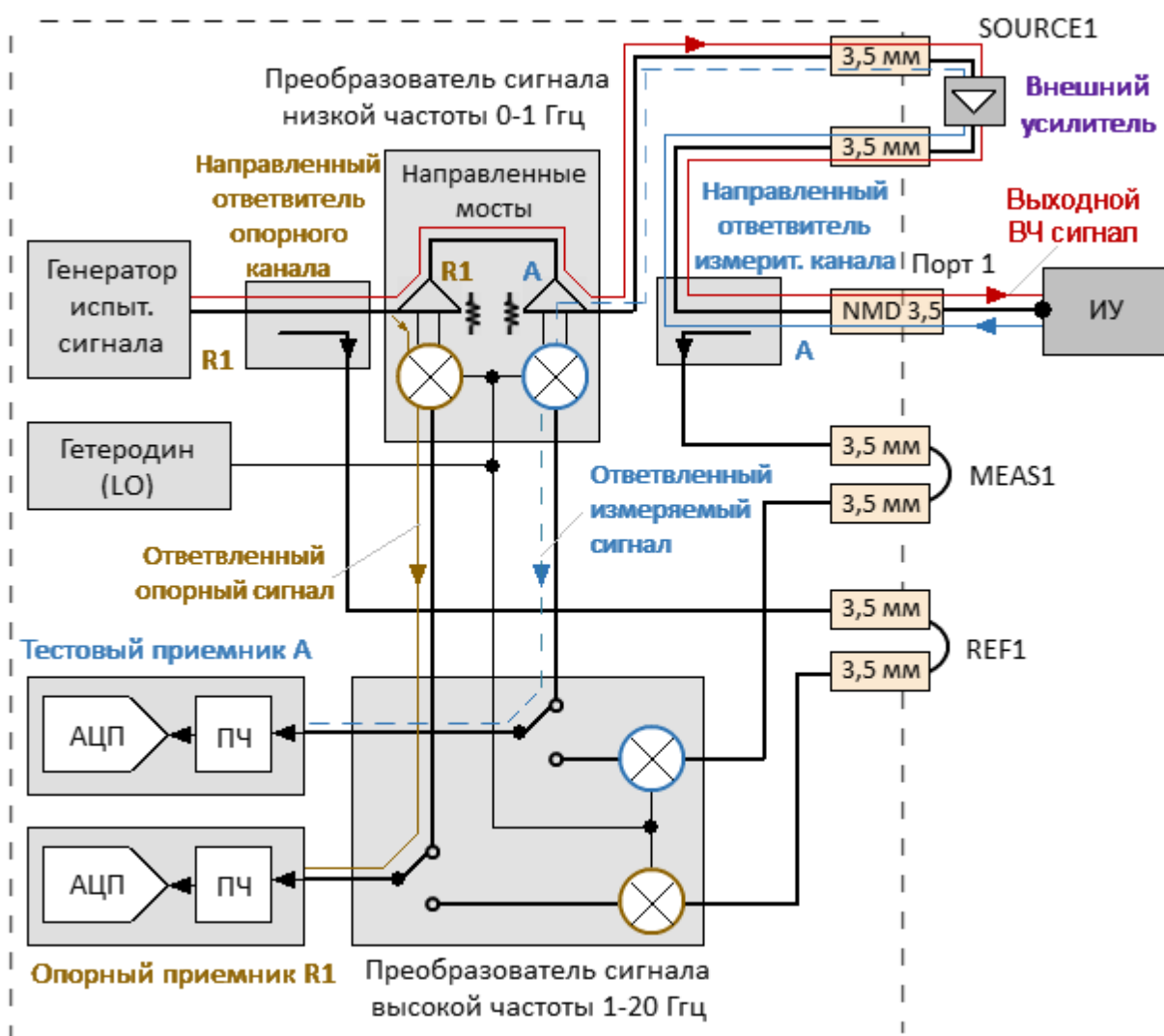
Рисунок 236 – Анализатор C2220, распространение сигнала с внешним усилителем в тракте генератора (диапазон от 100 кГц до 1 ГГц)
