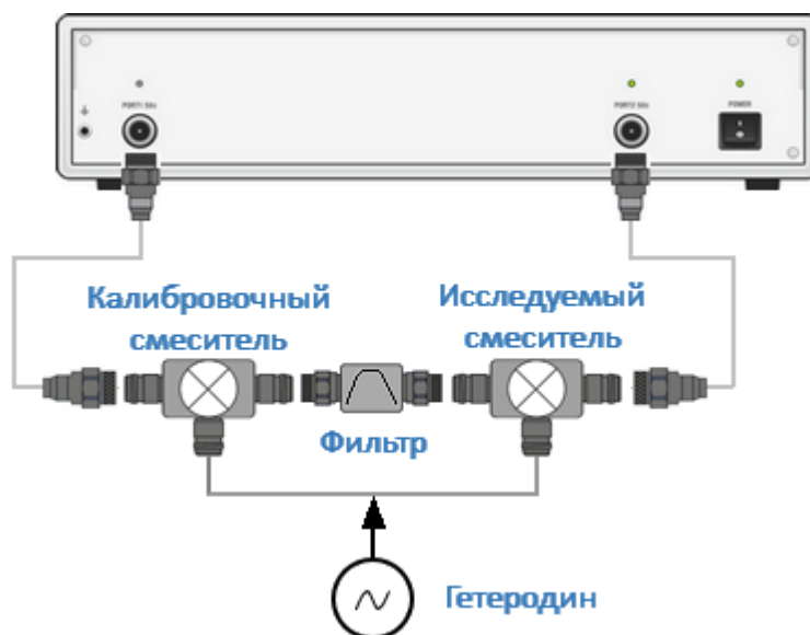
Рисунок 213 – Схема векторного измерения смесителя
