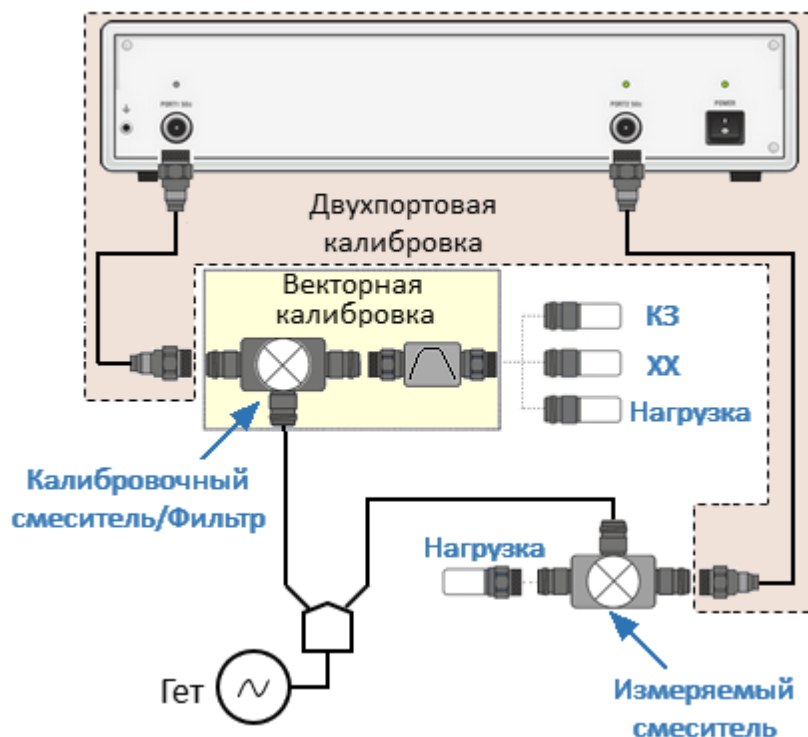
Рисунок 158 – Векторная калибровка смесителей
