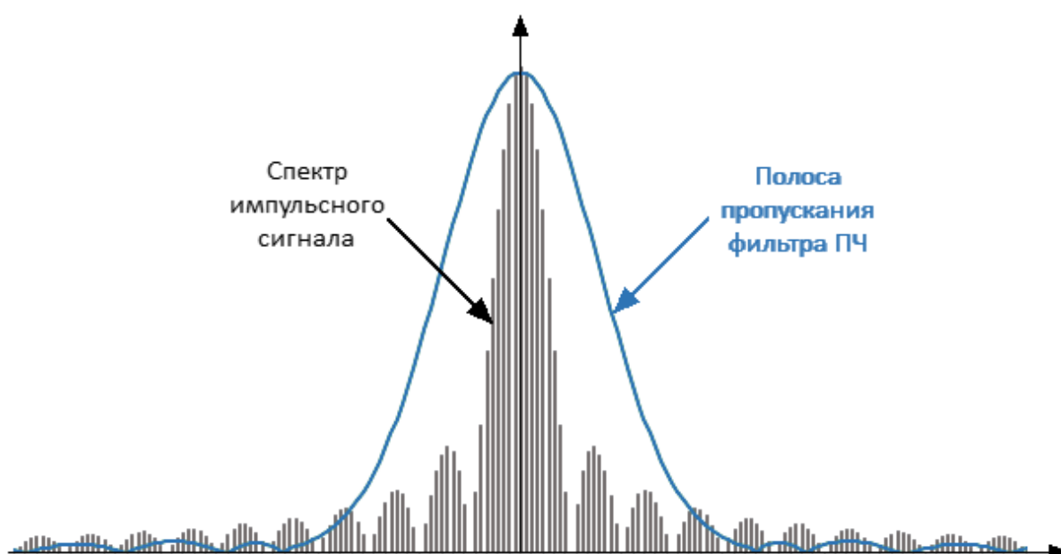
Рисунок 238 – Широкополосное детектирование
