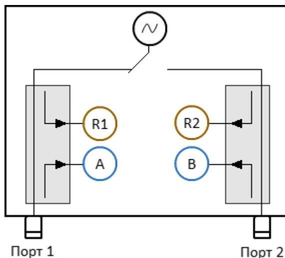
Рисунок 72 — Структурная схема анализатора
