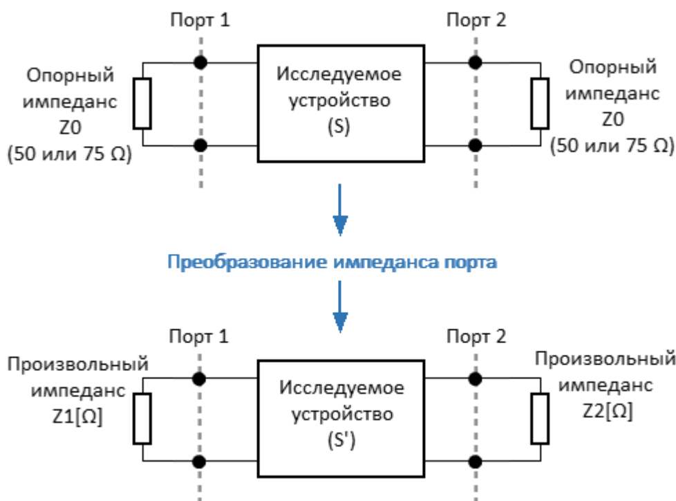
Рисунок 194 – Преобразование импеданса порта
