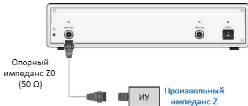
Рисунок 193 – Пример измерения анализатором с опорным импедансом 50 Ом ИУ с произвольным импедансом
