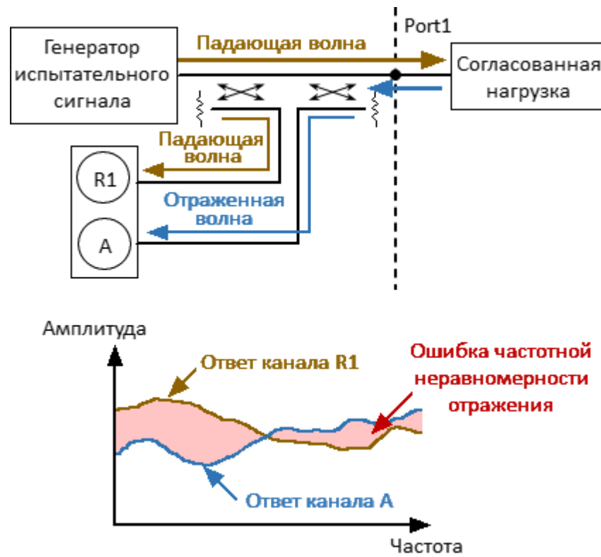
Рисунок 115 – Ошибка частотной неравномерности отражения
