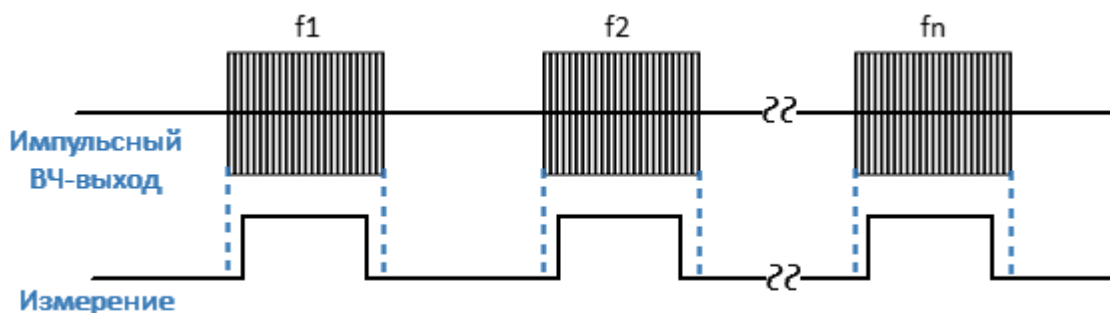
Рисунок 240 – Метод «Точка в импульсе»
