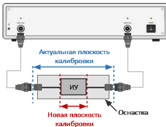
Рисунок 192 – Удлинение портов
