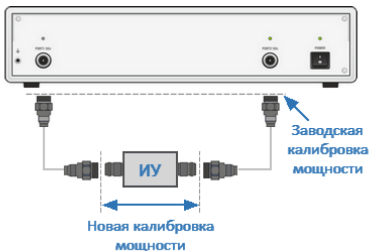
Рисунок 152 – Калибровка мощности
