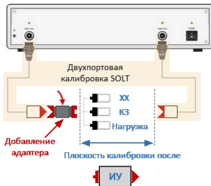
Рисунок 148 – Второй этап функции добавления адаптера
