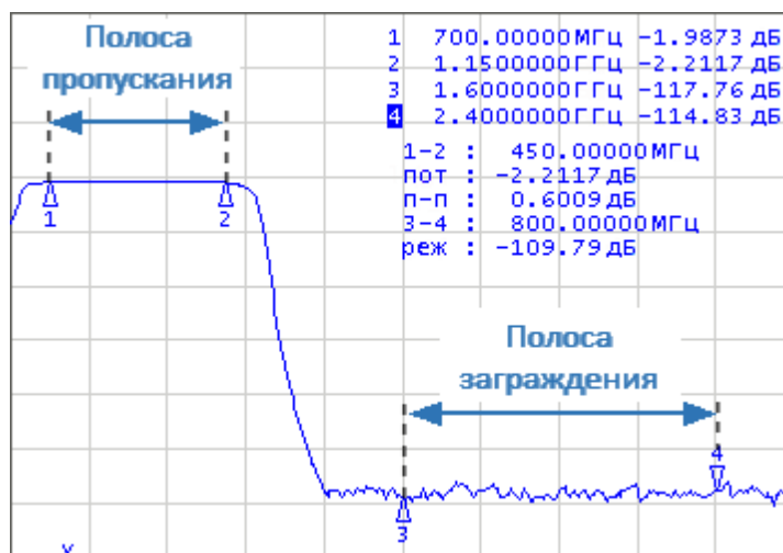
Рисунок 188 – Характеристики полосового фильтра
