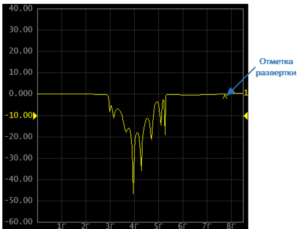
Рисунок 274 – Отметка развертки
