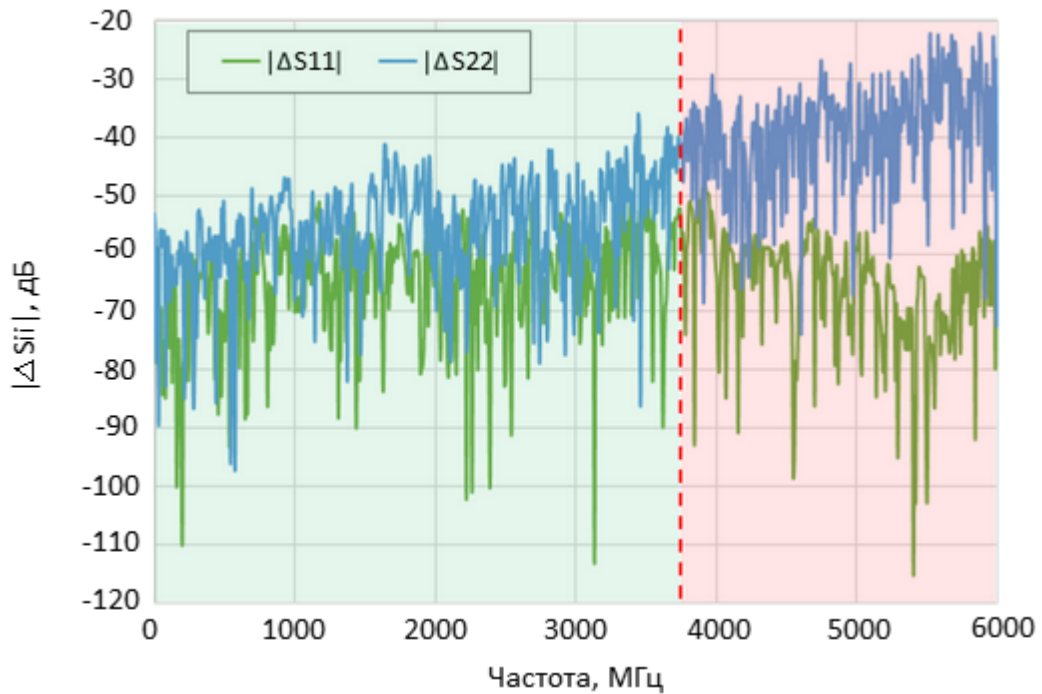
Рисунок 169 – Отклонение коэффициента отражения
